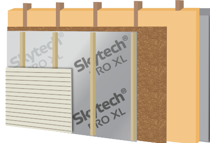
<중목구조> 중부2지역 총족
